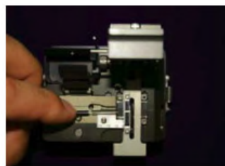
6. Leikkaa kuitu niin, että jäljelle jää 10 mm 125 µm:n kuidusta.
