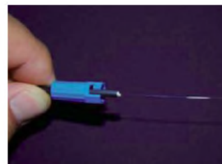
3. Kuori ulkovaippaa ja 900 µm:n päällystettä vähintään 50 mm:n matkalta
